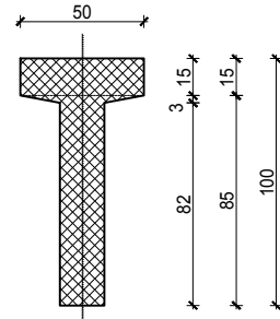
GLAVNI NOSAČ "T 100" pos GN10 R 1:50
