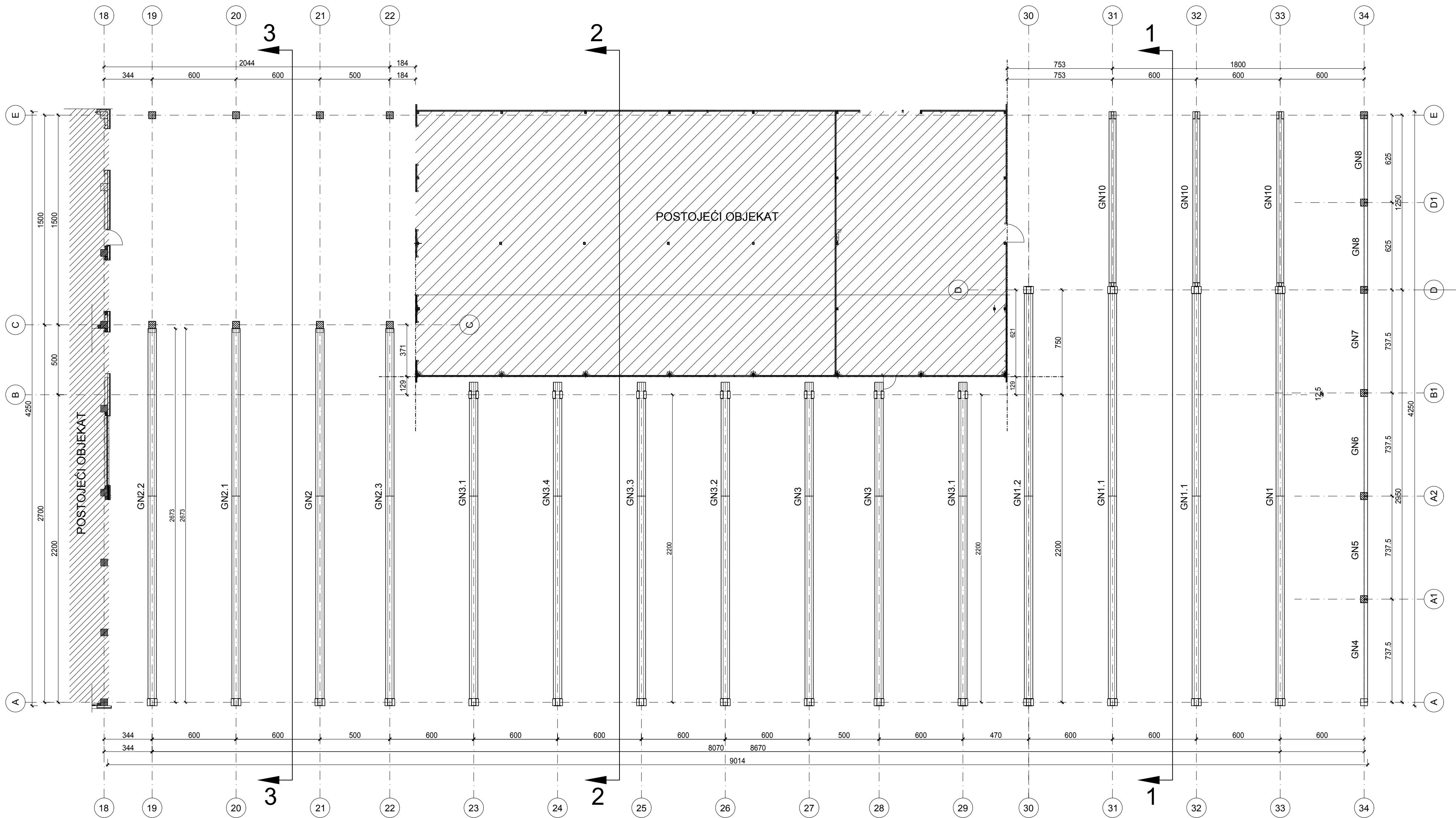
GLAVNI NOSAČ "A 145" pos GN1 - GN3.4 R 1:50
