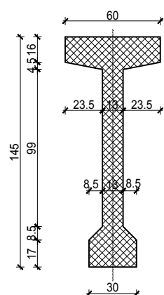
GLAVNI NOSAČ "A 145" pos GN1 - GN3.4 R 1:50
