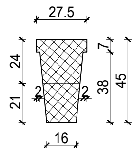
SEKUNDARNI NOSAČ "R 45" pos R1 - R7 R 1:50
