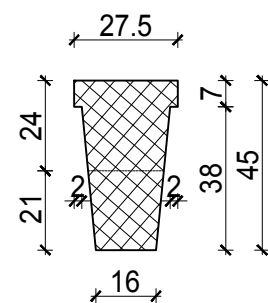
SEKUNDARNI NOSAČ "R 45" pos R7 R 1:50
