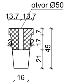
presek B-B R=1:25
